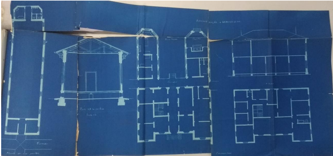
Figura 15 - Planta do Pavilhão Administrativo (primeira construção do novo complexo), 1903. 195
